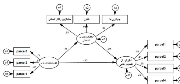
شکل ۲- ضرایب استاندارد شده مدل تحلیل معادلات ساختاری
