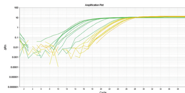
شکل ۷: منحنی تکثیر تصاعدی ژن‌های CXCL11 و B2M برحسب (سیکل-ΔRn) در بیماران مبتلا به سلپاک و افراد سالم.
