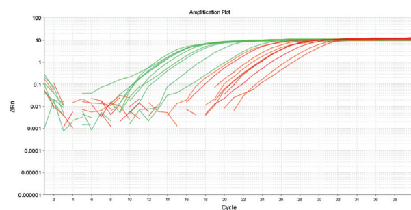
شکل ۶: منحنی تکثیر تصاعدی ژن‌های CXCL10 و B2M برحسب (سیکل-ΔRn) در بیماران مبتلا به سلپاک و افراد سالم.
