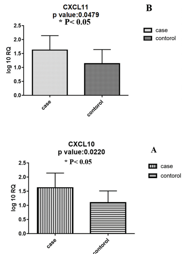
شکل ۸: میزان تغییرات بیان ژن‌های هدف در افراد مبتلا به سلپاک در مقایسه با افراد سالم. (A) تغییرات بیان ژن CXCL11 (B) تغییرات بیان ژن CXCL10.
